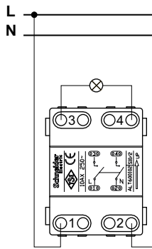
Двухполюсный выключатель
