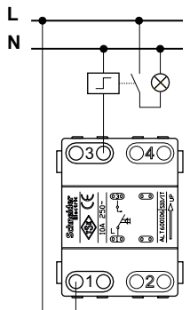
Кнопочный выключатель
