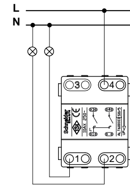
Двухклавишный выключатель
