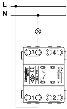
Одноклавишный выключатель
